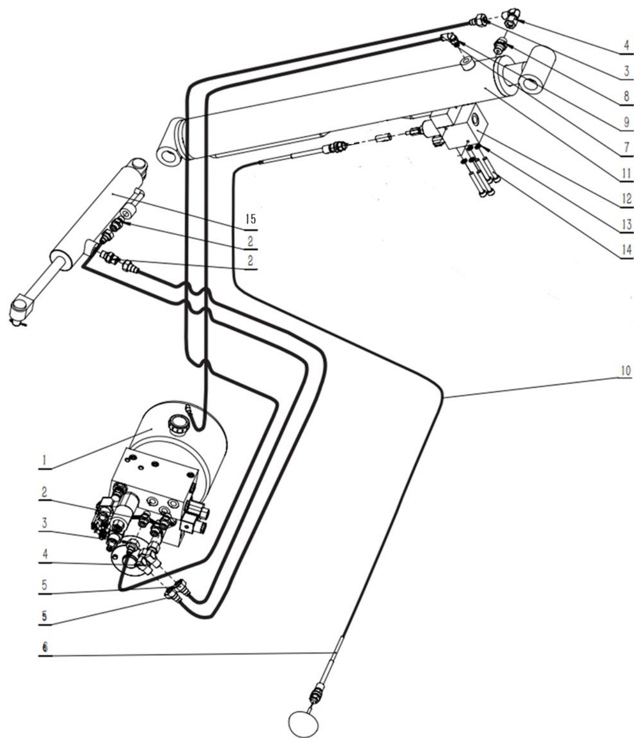
4-1 胶管连接示意图
