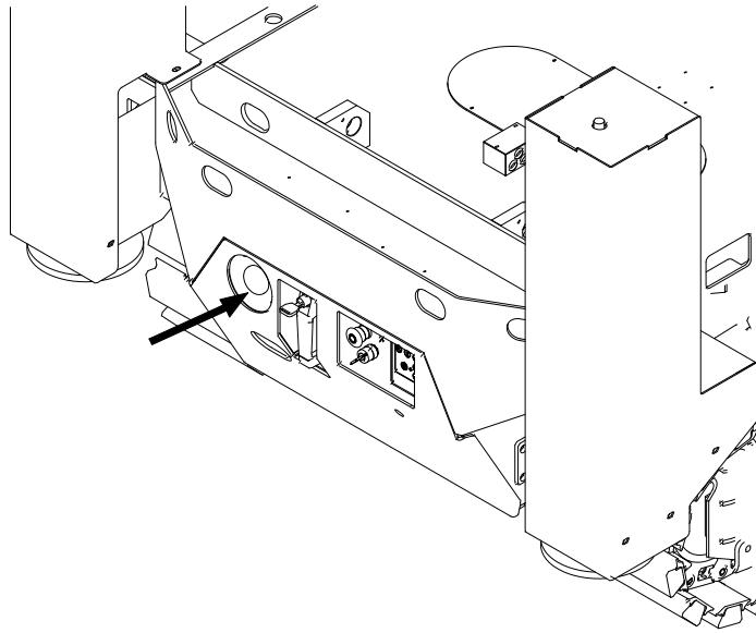
断电开关示意图
