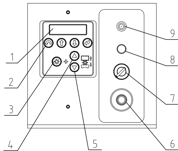
下控制面板
