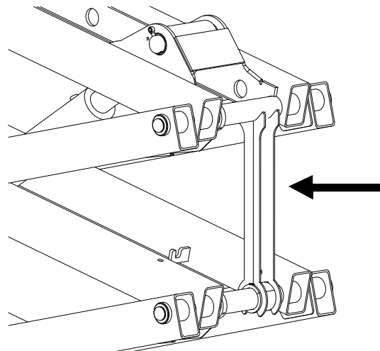
维修臂示意图
