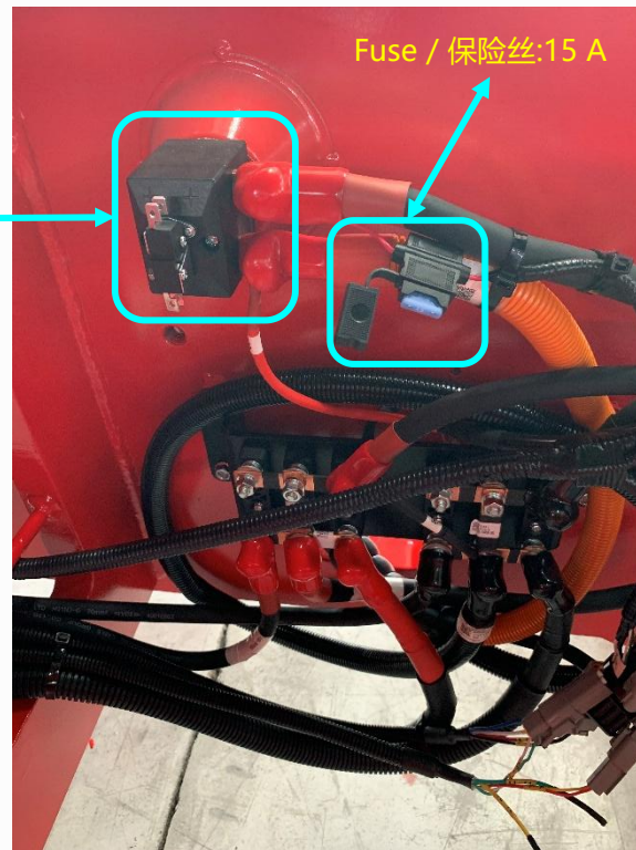
E-stop switch / 电源总开关
