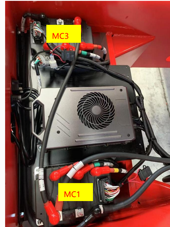
MC location / 控制器位置
