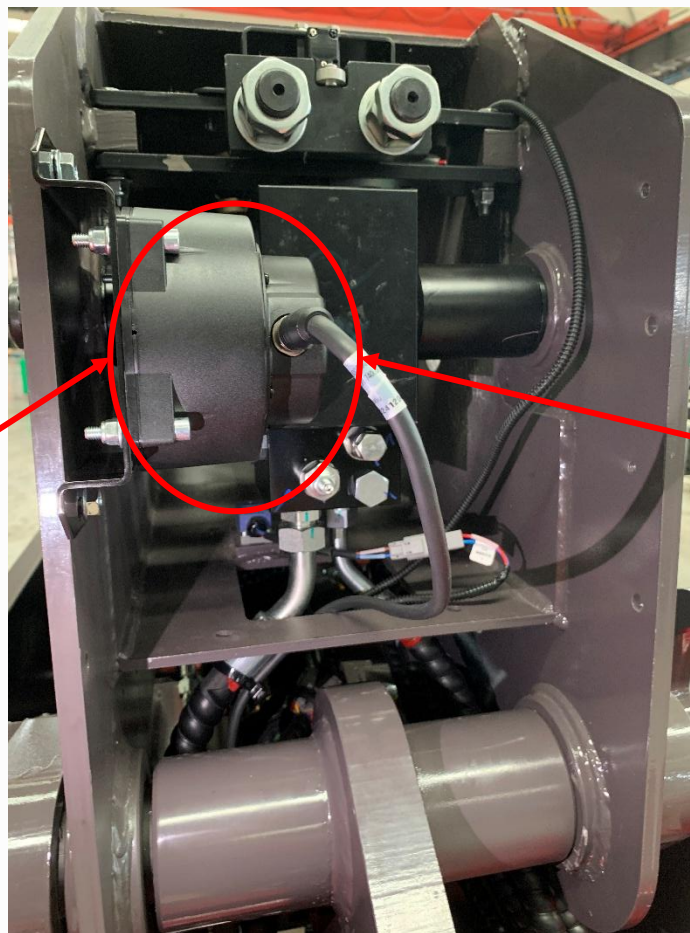
Length & Angle Sensor Location / 长角传感器位置
