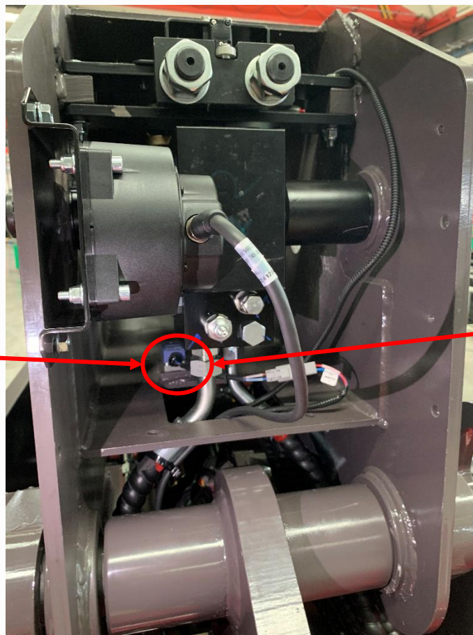
Boom retract Sensor Location / 全缩开关位置
