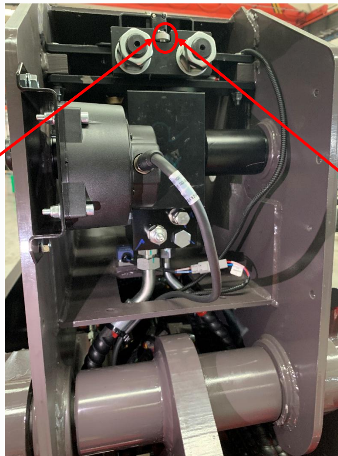
Boom steel cable sensor Diagram / 钢丝绳开关信号位置
